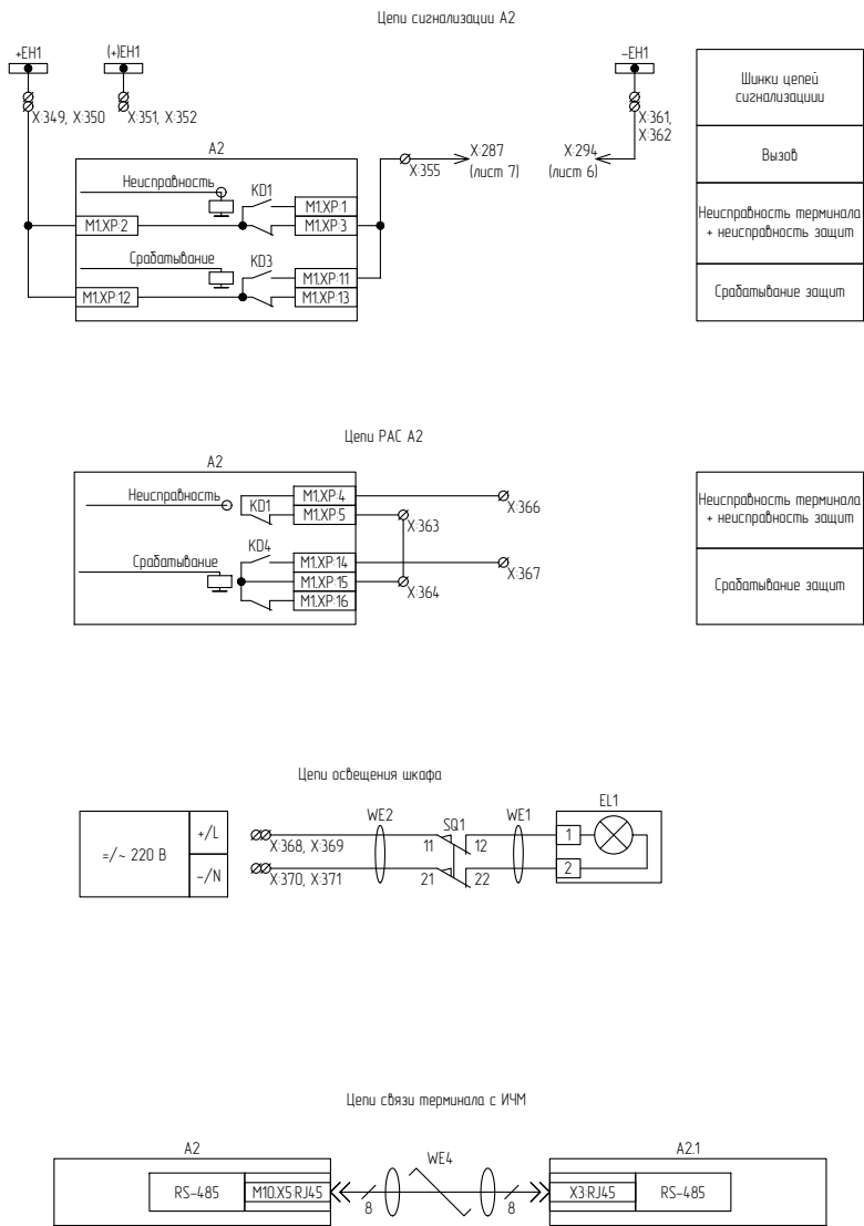
Рисунок Г.10 – Схема электрическая принципиальная (часть 10)
